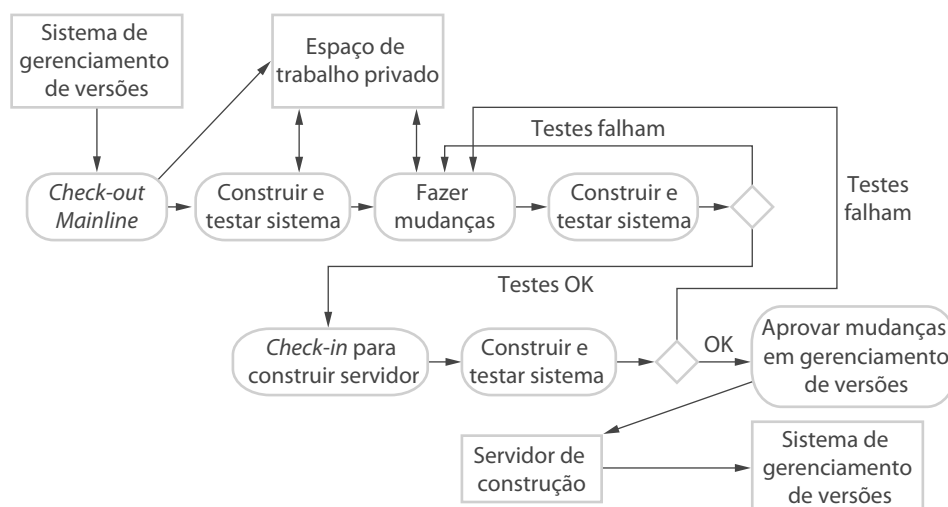
Figura 25.9 Integração contínua
